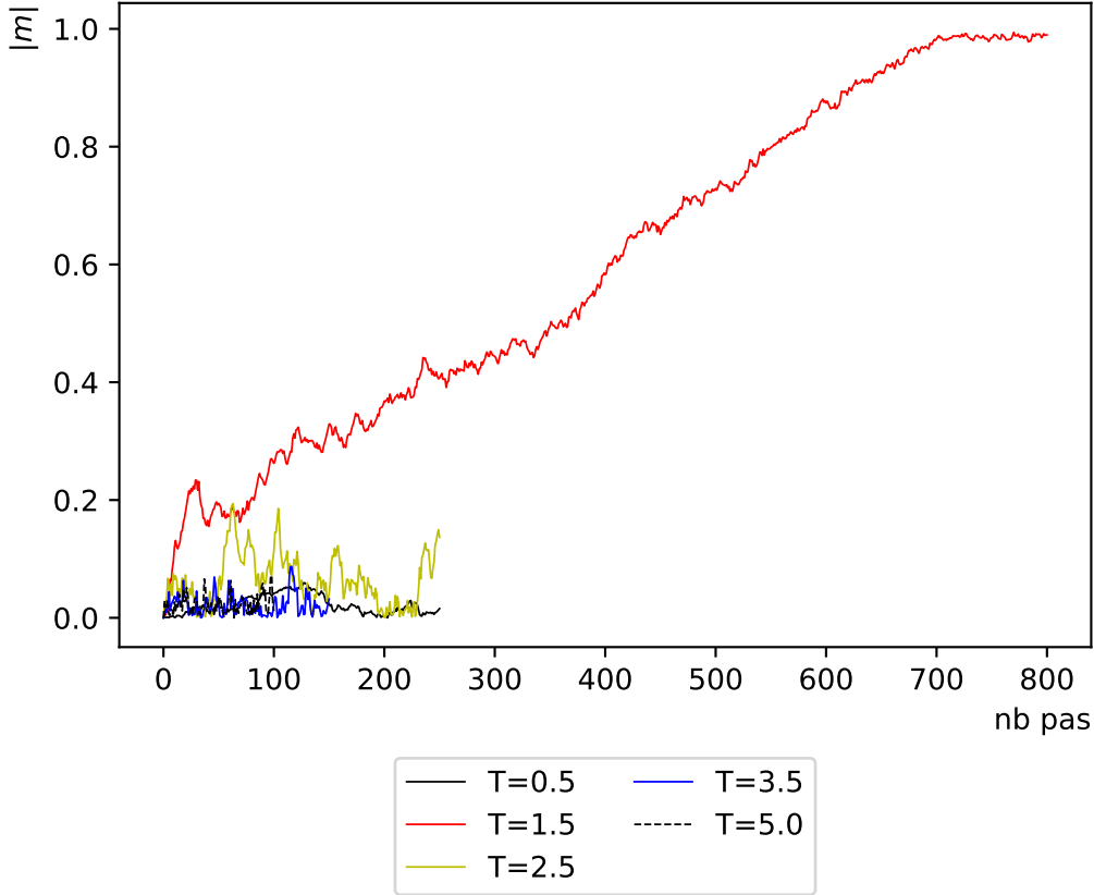
Evolution selon critère Estimation par intervalle,Condition Initiale alterné 4lignes-4lignes, Réseau taille L=64
